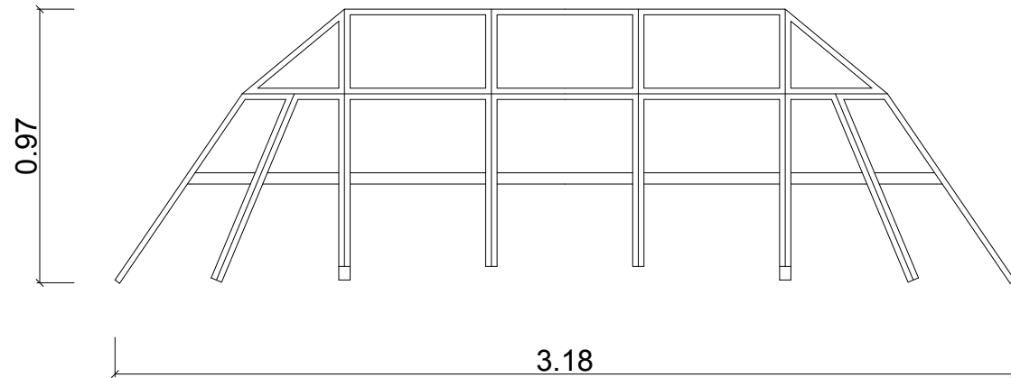
Vorderansicht
